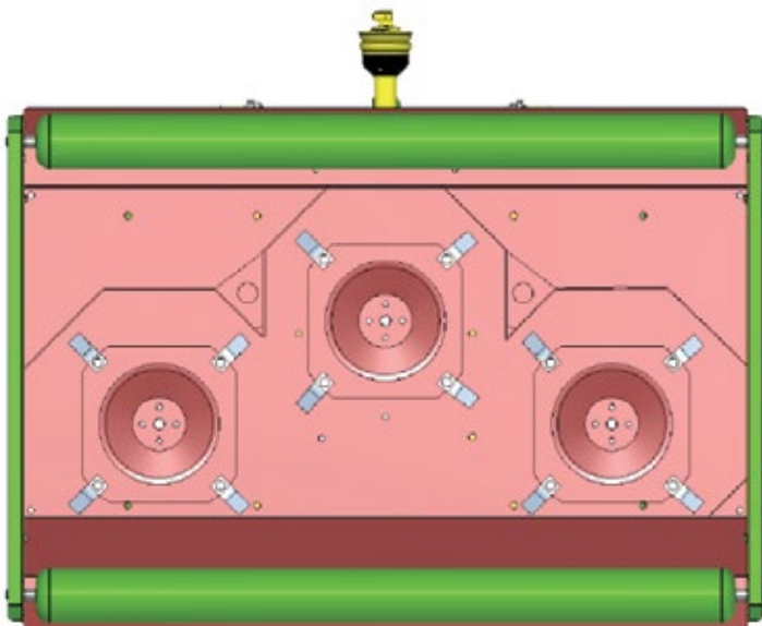
Die Falcon F210 Finishing Mower is toegerus met drie vierkantige, lae-impak-lemmskywe met vier spesiale gekrukte en ingekeepte lemme.
